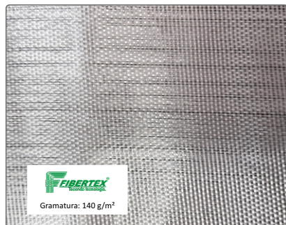
Artigo: AF – 0029 Desenho: Tela 1x1 Espessura: 0,13 mm Largura: 1300 mm
