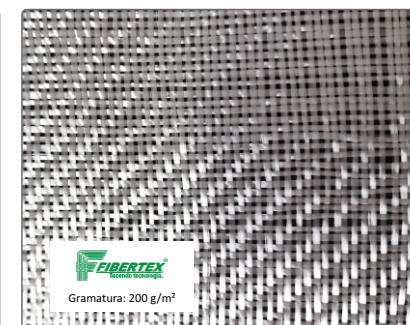
Artigo: AF – 0201 Desenho: Sarja 3x1 Espessura: 0,19 mm Largura: 1300 mm
