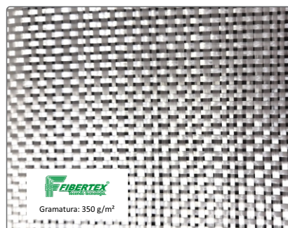
Artigo: AF – 0006 Desenho: Tela 1x1 Espessura: 0,40 mm Largura: 650 mm
