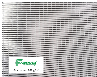
Artigo: UF – 0363 Sentido: Transversal Espessura: 0,85 mm Largura: 1400 mm
