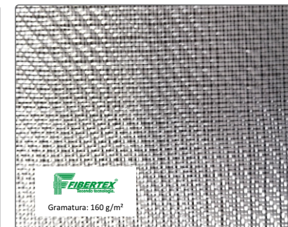
Artigo: AF – 0016 Desenho: Sarja 3x1 Espessura: 0,18 mm Largura: 1300 mm
