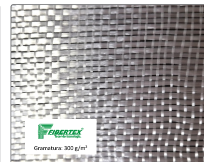
Artigo: AF – 0300 Desenho: Tela 1x1 Espessura: 0,28 mm Largura: 1300 mm
