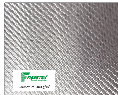
Artigo: AF – 0299 Desenho: Sarja 2x2 Espessura: 0,21 mm Largura: 1300 mm
