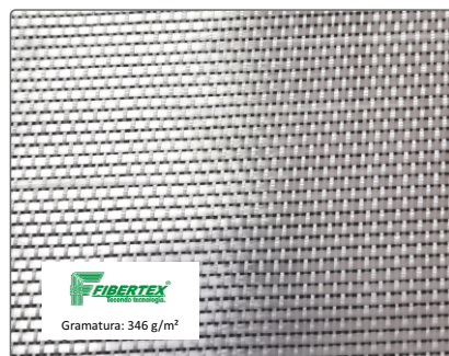
Artigo: UF – 0346 Sentido: Transversal Espessura: 0,45 mm Largura: 1300 mm
