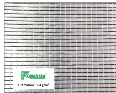
Artigo: UF – 0595 Sentido: Transversal Espessura: 0,85 mm Largura: 1800 mm
