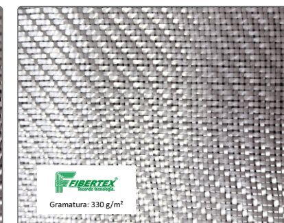
Artigo: AF – 0330 Desenho: Sarja 3x1 Espessura: 0,30 mm Largura: 1300 mm
