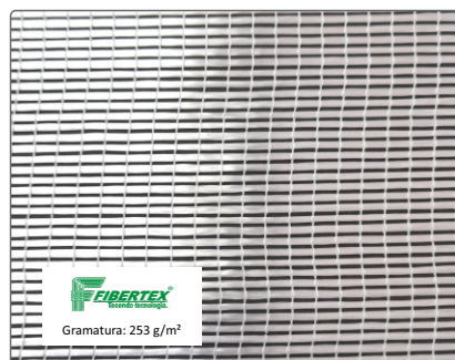
Artigo: UF – 0259 Sentido: Transversal Espessura: 0,30 mm Largura: 1250 mm
