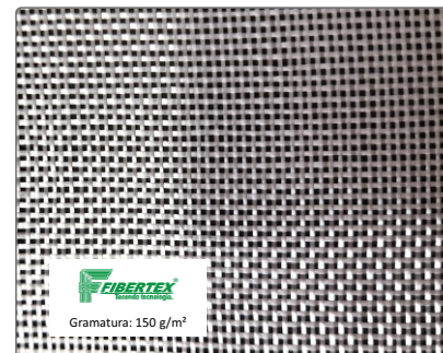
Artigo: AF – 0170 Desenho: Tela 1x1 Espessura: 0,16 mm Largura: 1300 mm
