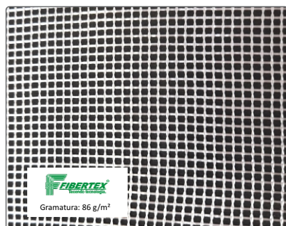
Artigo: AF – 0086 Desenho: Giro Inglês Espessura: 0,15 mm Largura: 1430 mm
