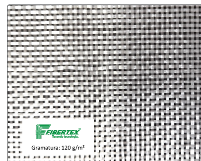
Artigo: AF – 0012 Desenho: Tela 1x1 Espessura: 0,13 mm Largura: 1300 mm
