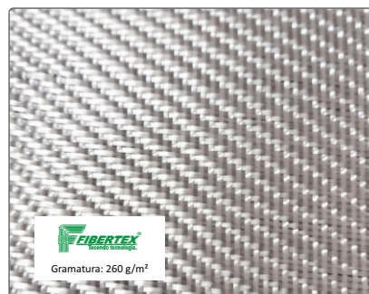
Artigo: AF – 0260 Desenho: Sarja 3x1 Espessura: 0,23 mm Largura: 1300 mm
