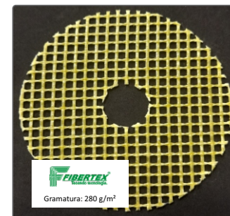
Artigo: AF – 0251 Desenho: Giro Inglês Gramatura: 280 g/m 2 Espessura: 0,65 mm Abertura de Malha: 2x2mm
