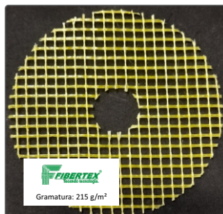
Artigo: AF – 0200 Desenho: Giro Inglês Gramatura: 215 g/m 2 Espessura: 0,50 mm Abertura de Malha: 5x5mm
