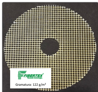
Artigo: AF – 0086 Desenho: Giro Inglês Gramatura: 122 g/m 2 Espessura: 0,30 mm Abertura de Malha: 2x2mm
