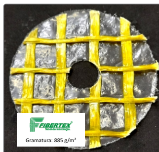
Artigo: AF – 0601 Desenho: Tela Gramatura: 885 g/m 2 Espessura: 1,22 mm Abertura de Malha: 16x21mm
