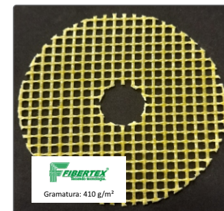
Artigo: AF – 0380 Desenho: Giro Inglês Gramatura: 410 g/m 2 Espessura: 0,90 mm Abertura de Malha: 5x5mm
