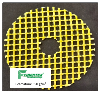
Artigo: AF – 0470 Desenho: Giro Inglês Gramatura: 550 g/m 2 Espessura: 2,20 mm Abertura de Malha: 5x5mm
