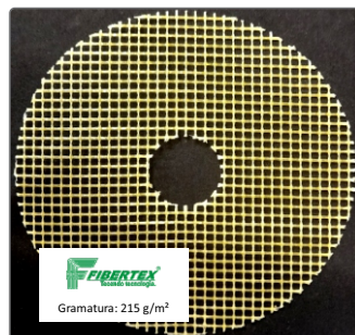
Artigo: AF – 0187 Desenho: Giro Inglês Gramatura: 215 g/m 2 Espessura: 0,40 mm Abertura de Malha: 2x2mm
