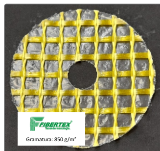
Artigo: AF – 0680 Desenho: Giro Inglês Gramatura: 850 g/m 2 Espessura: 1,25 mm Abertura de Malha: 10x10mm
